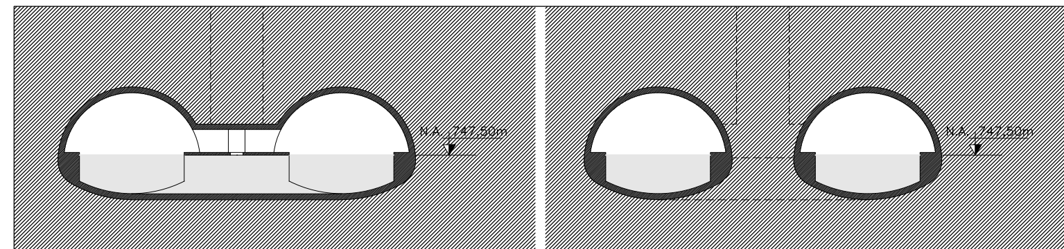
TÚNEL CANAL SEÇÃO VASO-COMUNICANTE TÚNEL CANAL SEÇÃO TIPO 1:500
